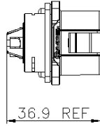
LP-24-J__SX-XX-001 Socket
