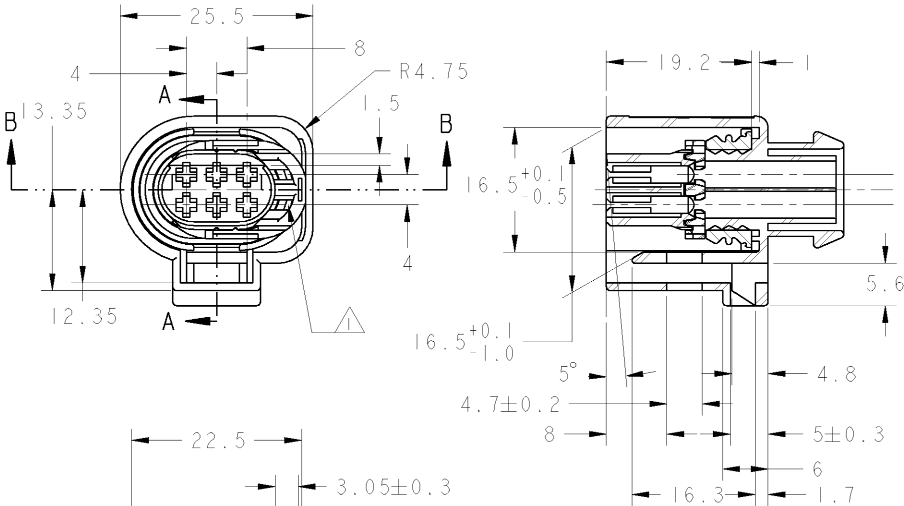
SECTION A-A
