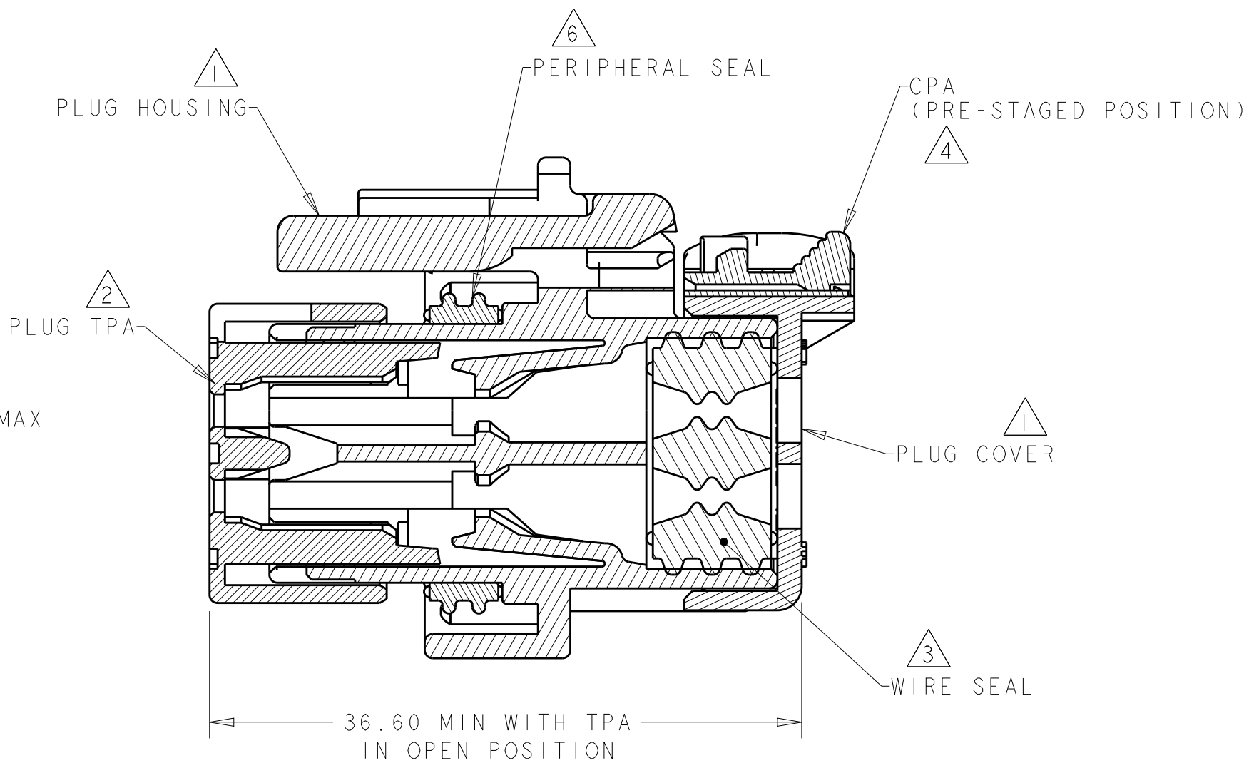
SECTION A-A
