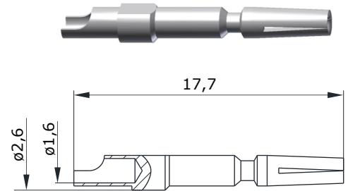
Hauptabmessungen Kontaktbuchse
