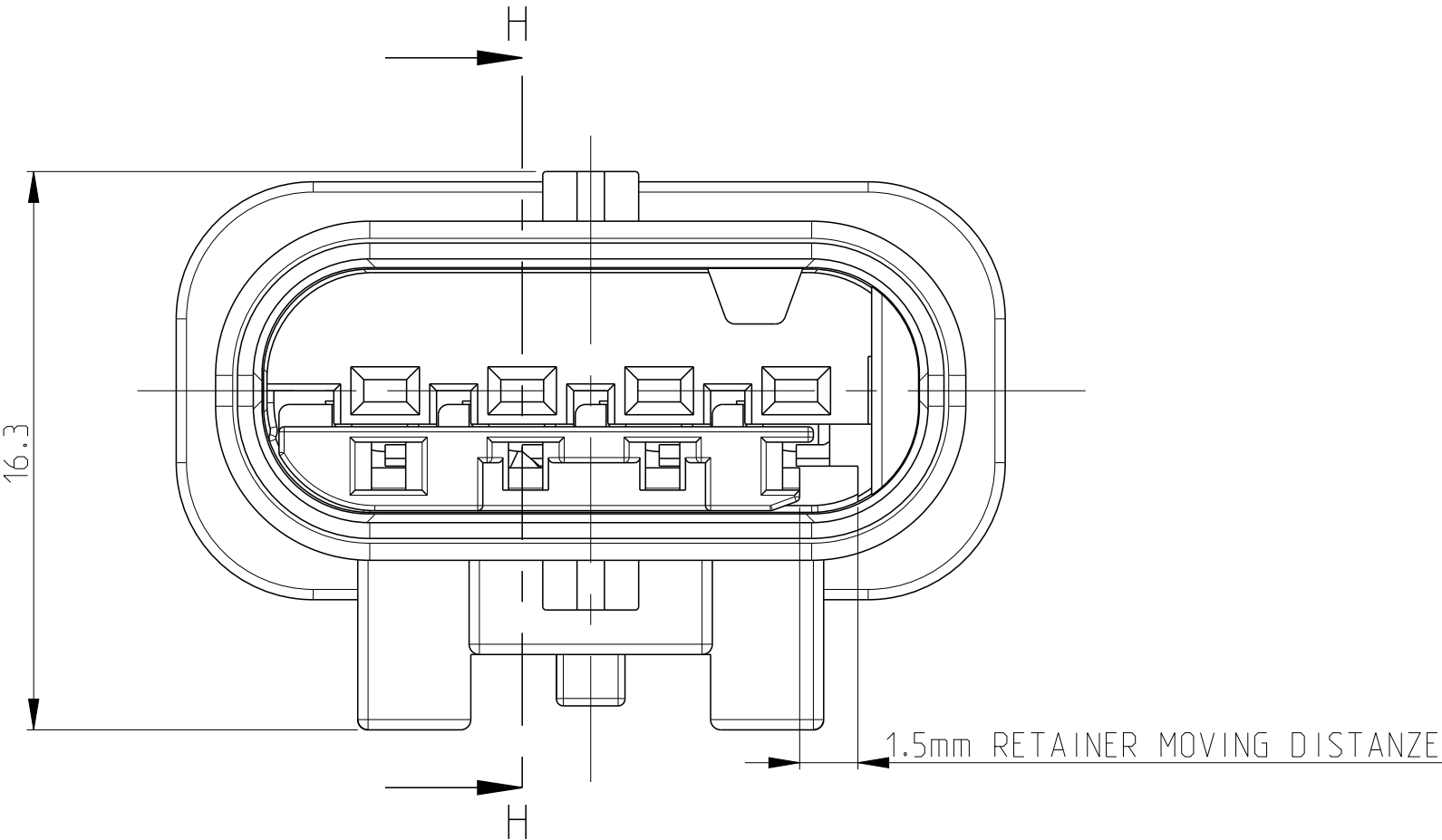
RETAINER IN FINAL LOCKED POSITION 2. Kontaktsicherung in Endraststellung
