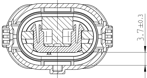
2-Kontaktsicherung in Endraststellung
