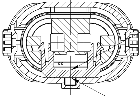
9 2-Kontaktsicherung in Vorraststellung
