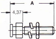
Schraubensatz 2-56 2-56 Locking Post Assembly
